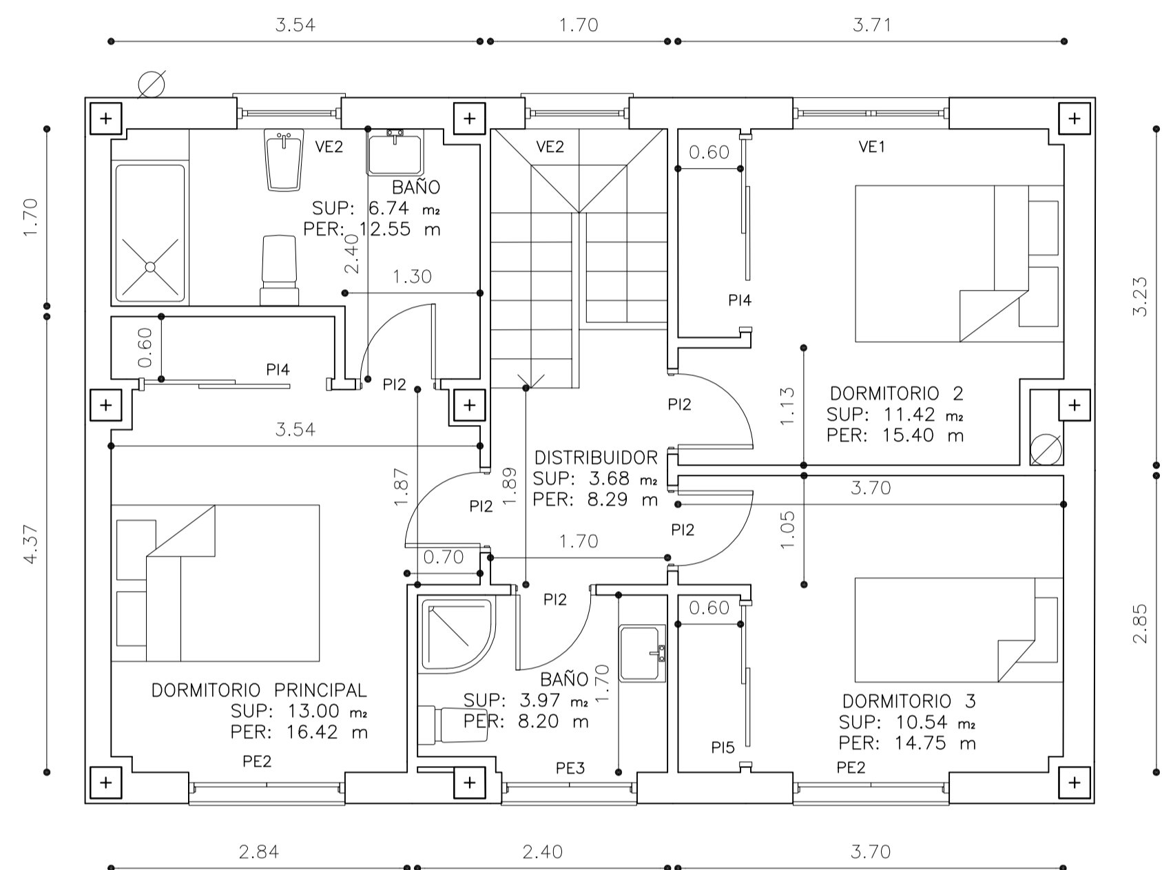
PLANTA PRIMERA
