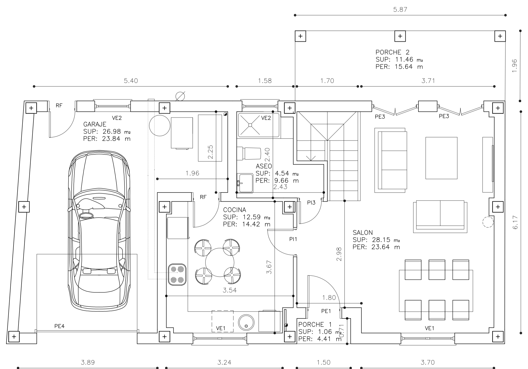
PLANTA BAJA
